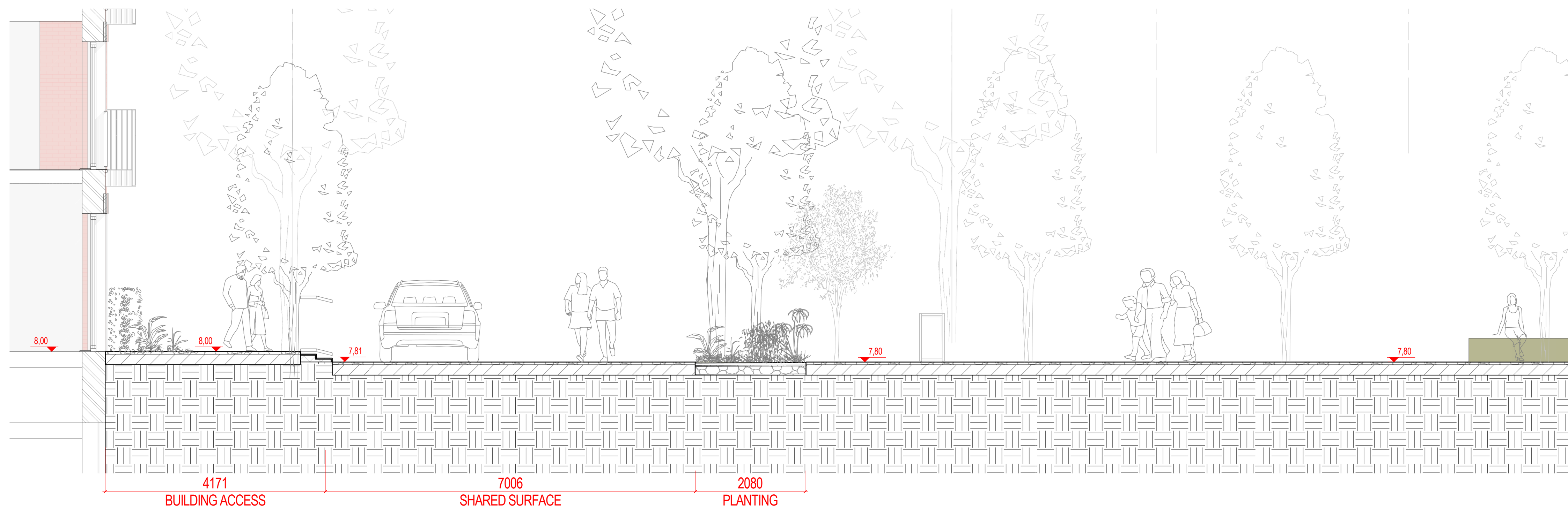
2 SECTION 43 1:50 @A1
