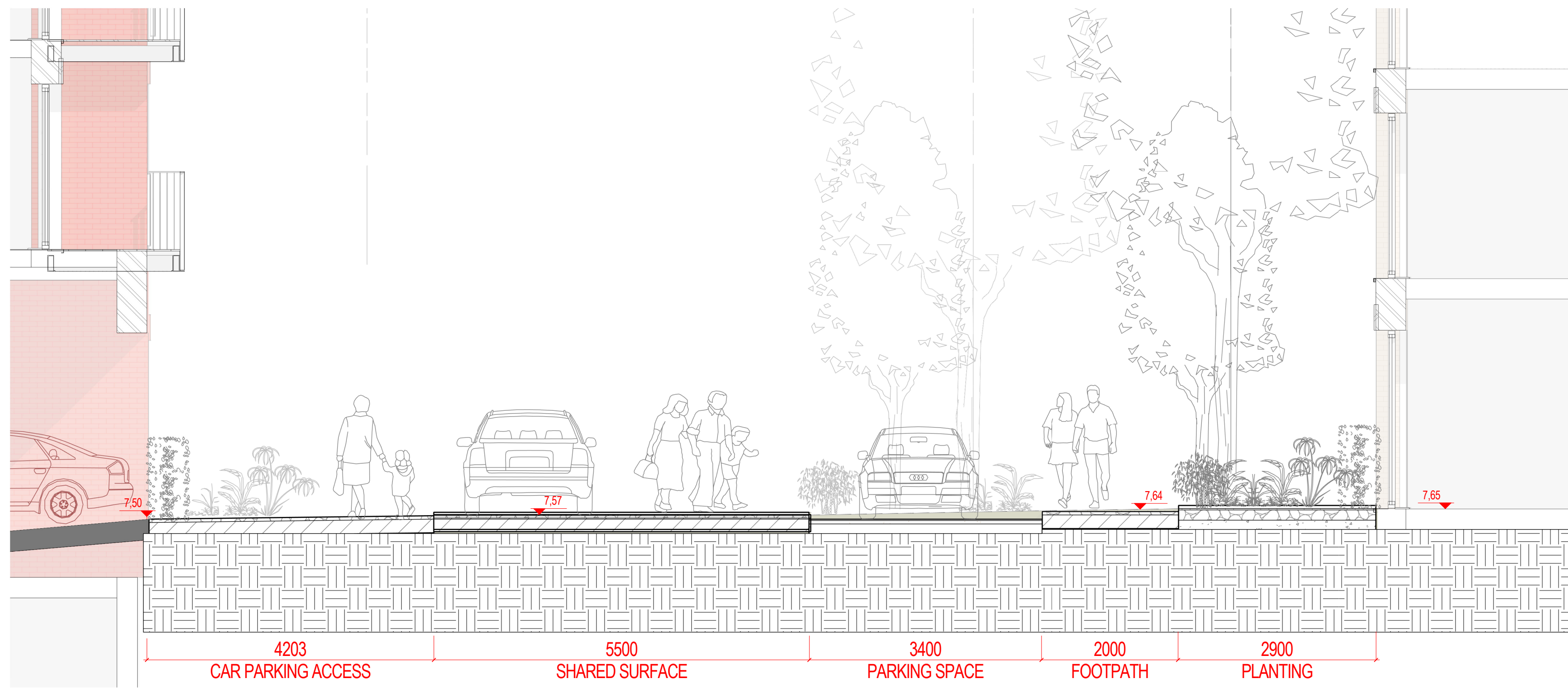
1 SECTION 42 1:50 @A1
